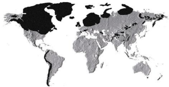
De globale verspreiding van het landijs op het hoogtepunt van de ijstijd. Naar: Mountain High Maps © www.Digiwis.com
